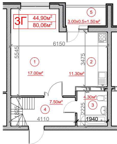
План 1 рівня квартири
