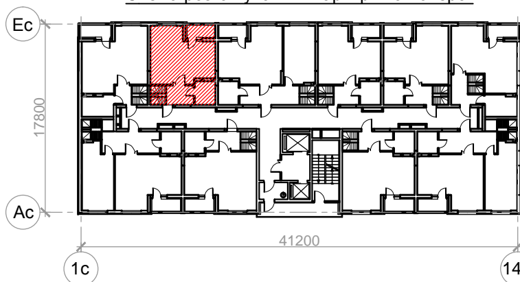
Схема розташування квартири на поверсі
